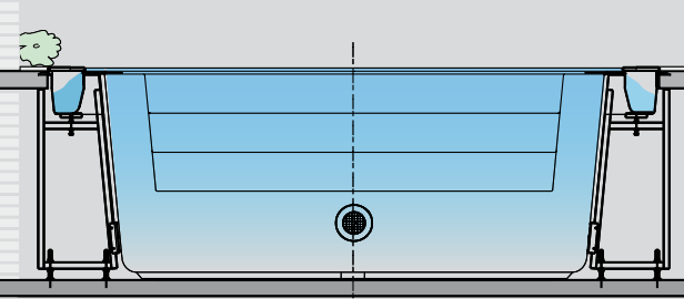
Einbau freitragend mit Überlaufrinne: Wandverstreibungen aus Stahl.
