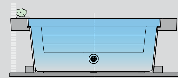
Einbau als freitragende Variante: Wandverstreibungen anlaminiert.
